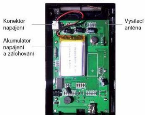
Pohled po odejmutí zadního krytu
